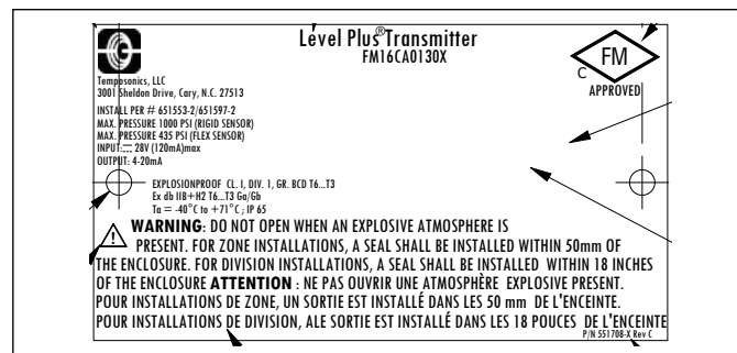
图 44: 防爆型, FMC 标签, HART®, 外壳选型 D、E
