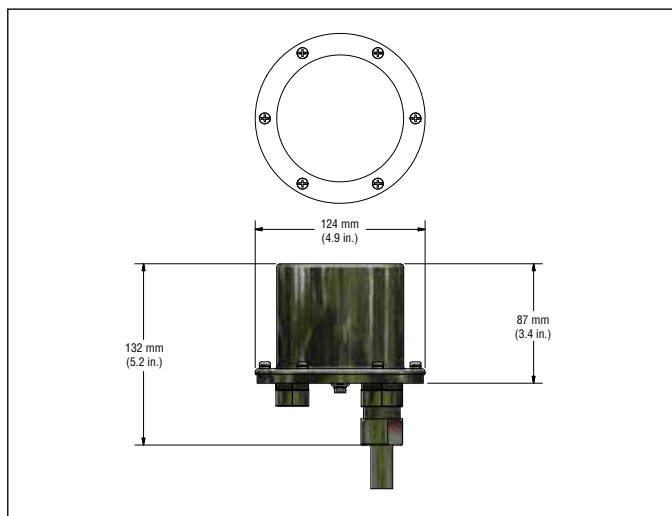
图 1: NEMA Type 4X 316L 不锈钢外壳
