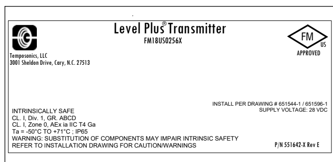
图 18: 本质安全型 FM 标签, HART®, 单腔或双腔外壳
