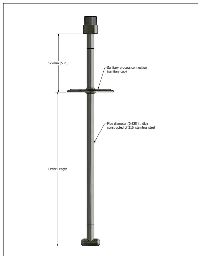
图 5: 外管配置
