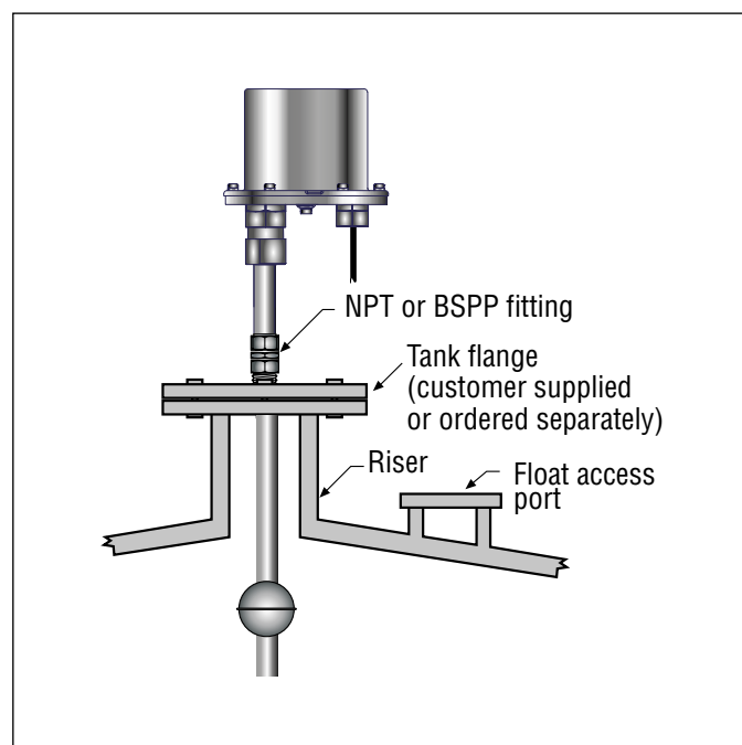
图 8: 挠性管的螺纹法兰安装
