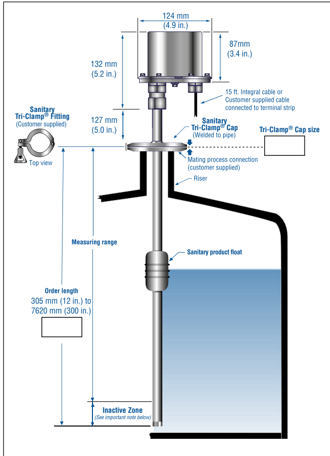
图 9: 管子三夹头安装
