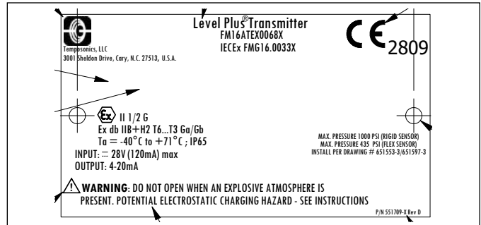
图 60: 防火型, ATEX 和 IECEx 标签, HART®, 外壳选型 D、E、G、H 或 L
