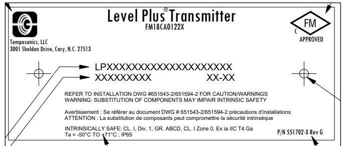
图 33: 本质安全型 FMC 标签, Modbus 和 DDA, 单腔或双腔外壳
