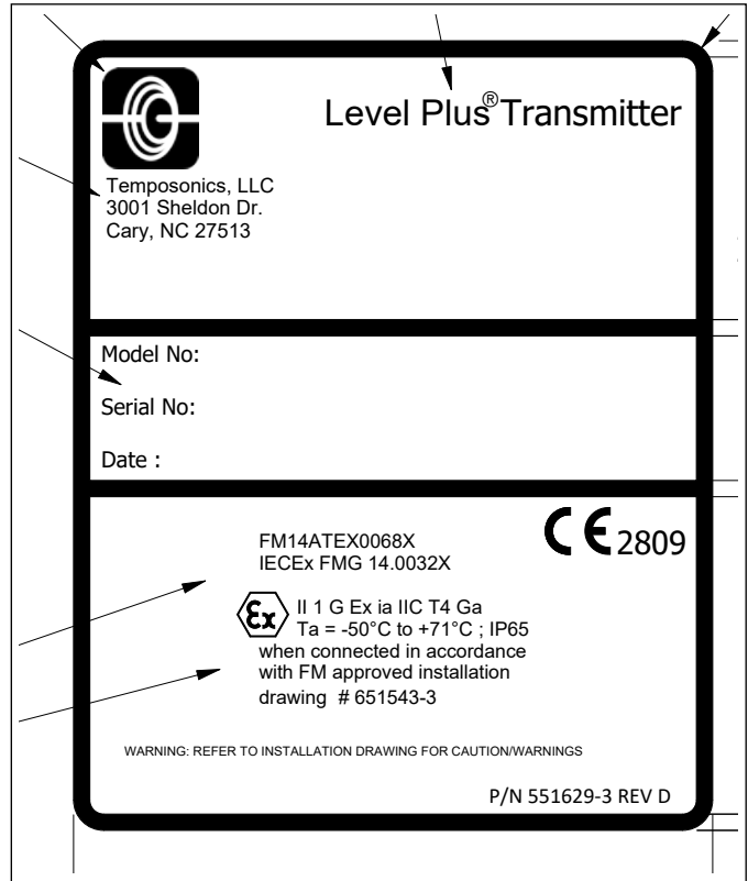
图 51: 本质安全型 FMC 标签, Modbus 和 DDA, NEMA 外壳
