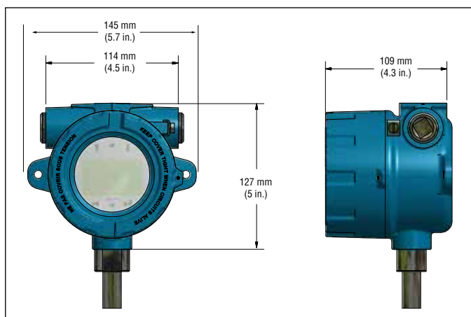
图 2: 单腔外壳
