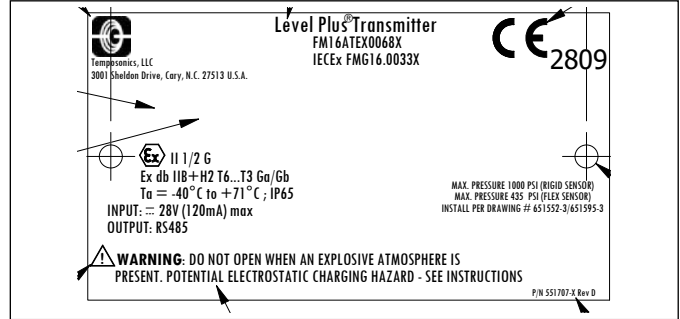
图 59: 防火型, ATEX 和 IECEx 标签, Modbus 或 DDA 外壳选型 D、E、G、H 或 L
