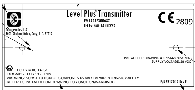
图 54: 本质安全型 ATEX/IECEX 标签, Modbus 和 DDA, 单腔或双腔外壳
