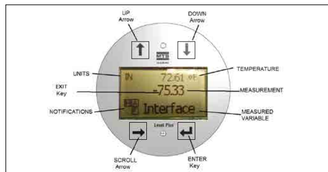
图1：显示器
