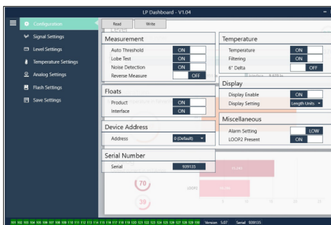
图5：通过配置表可针对特定应用配置液位变送器。
