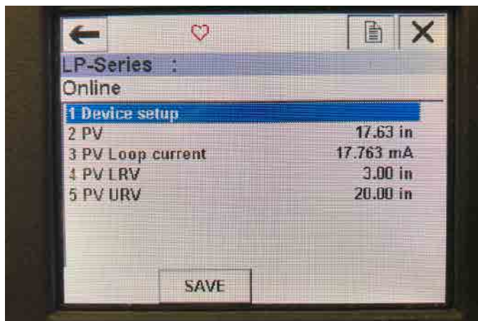
图12: 在线画面
