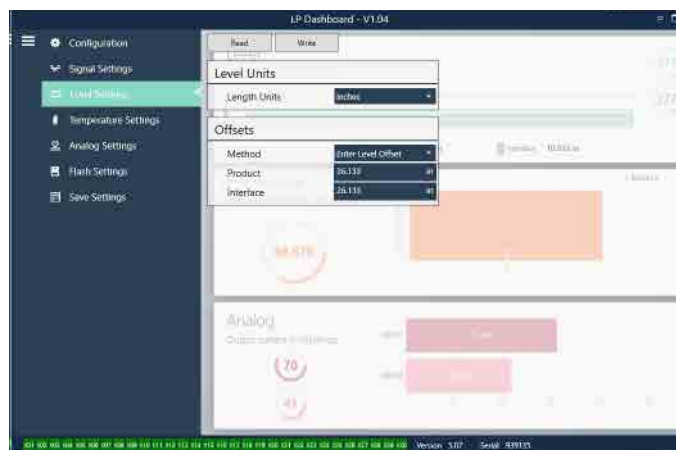
图7：液位设置
