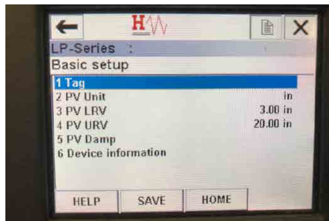
图23 : Basic setup (基本设置) 菜单画面
