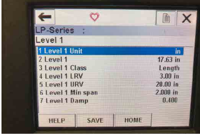
图31 : Level 1 (液位1) 菜单画面
