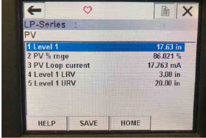
图16 : PV菜单树
