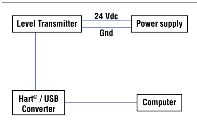
图2：安装实例
