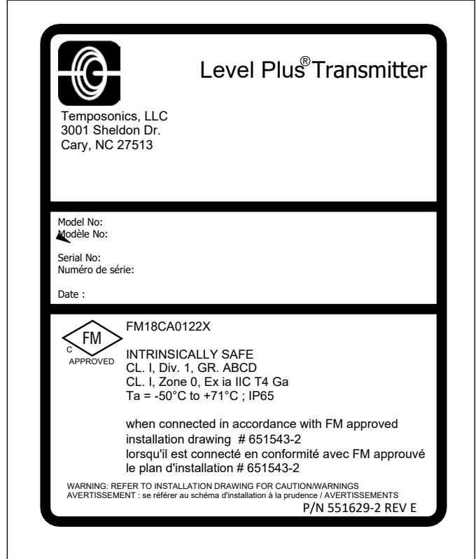
그림34: 본질 안전 FMC 라벨, Modbus 및 DDA, NEMA 하우징
