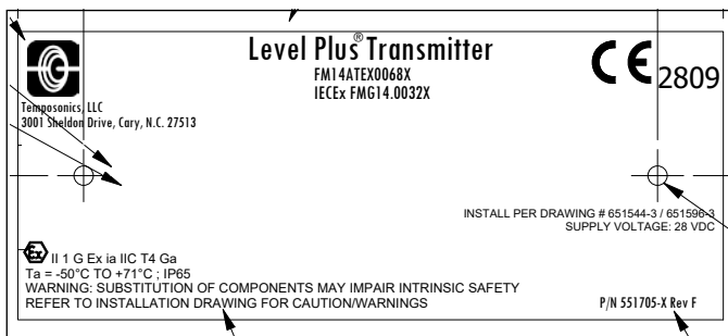
그림57: 본질 안전 ATEX/IECEX 라벨, Modbus 및 DDA, 단일 및 듀얼 캐비티 하우징
