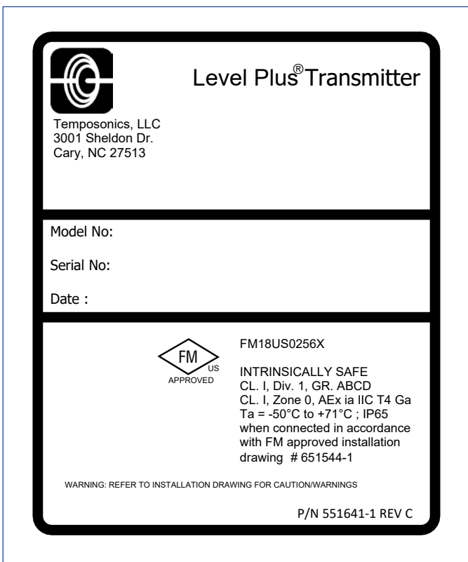
그림19: 본질 안전 FM 라벨, HART®, NEMA 하우징
