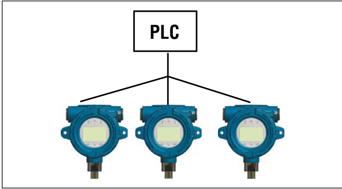
그림15: 트리 토폴로지
