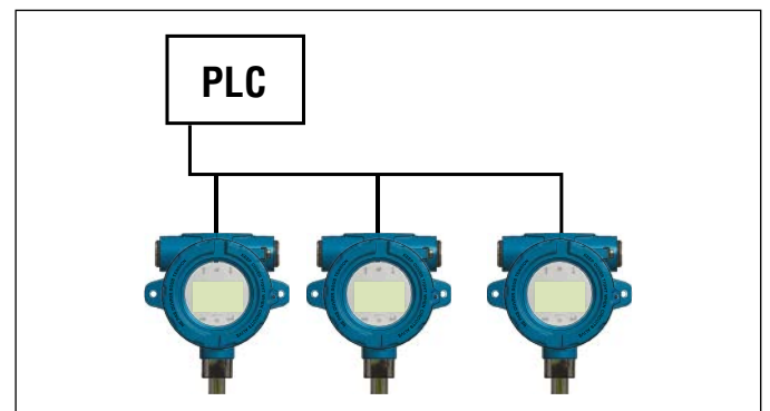
그림14: 스퍼 토폴로지 사용 버스
