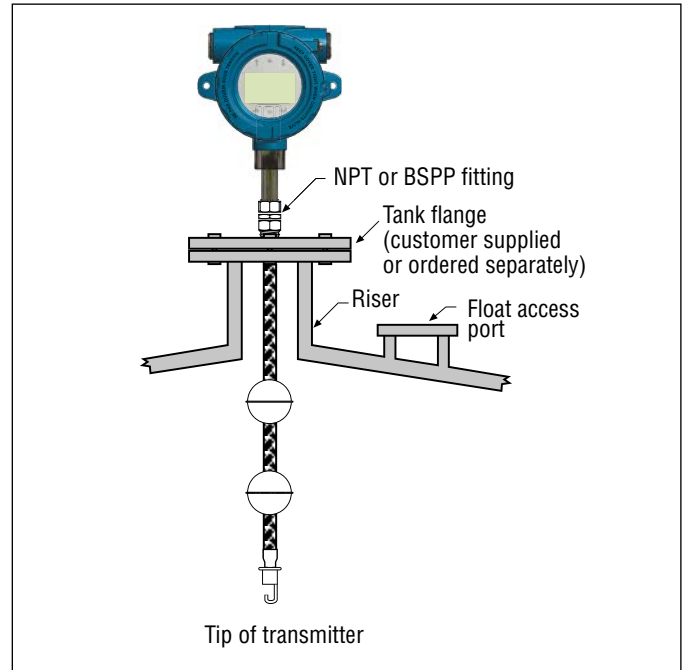
그림11: 플렉시블 파이프에 대한 스레드 플랜지 장착
