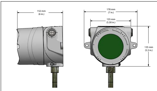
그림4: 스테인리스 스틸 단일 캐비티 하우징
