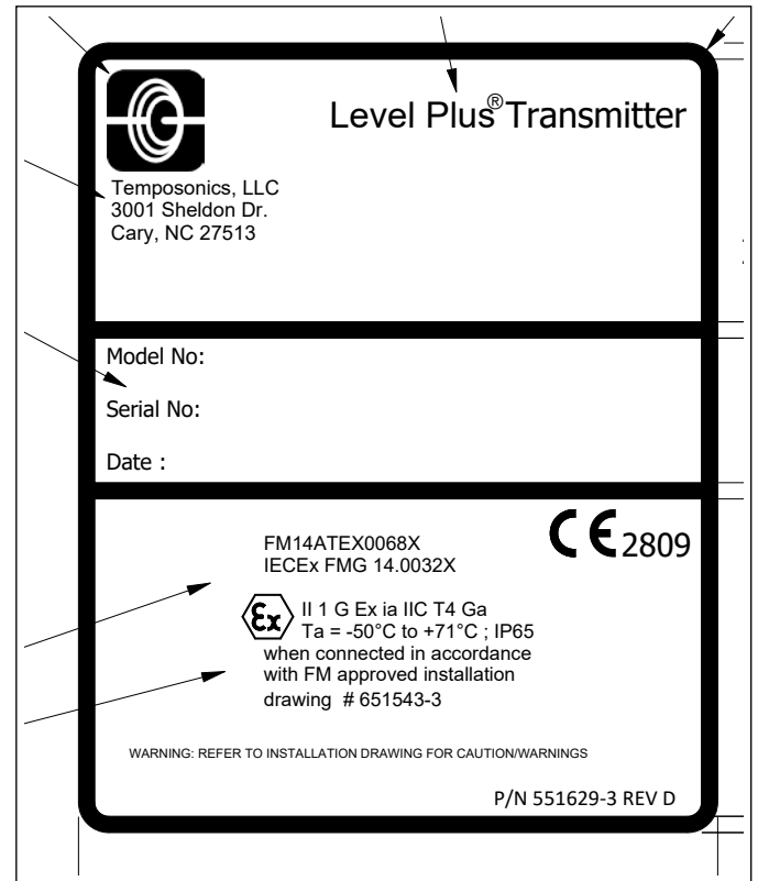
그림54: 본질 안전 FMC 라벨, Modbus 및 DDA, NEMA 하우징
