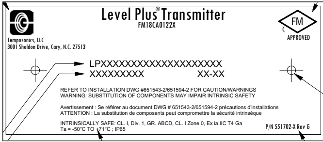
그림36: 본질 안전 FMC 라벨, Modbus 및 DDA, 단일 및 듀얼 캐비티 하우징
