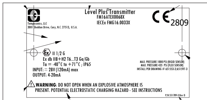
Fig. 60: À prova de chamas, etiqueta ATEX e IECEx, invólucro HART®, opções D, E, G, H ou L
