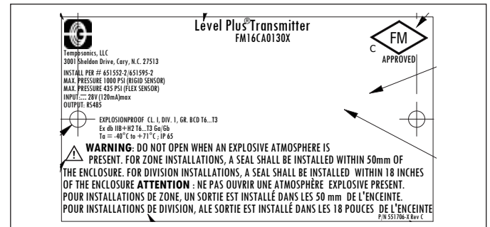
Fig. 41: À prova de explosão, etiqueta FMC, Modbus ou DDA, invólucro opções G, H ou L
