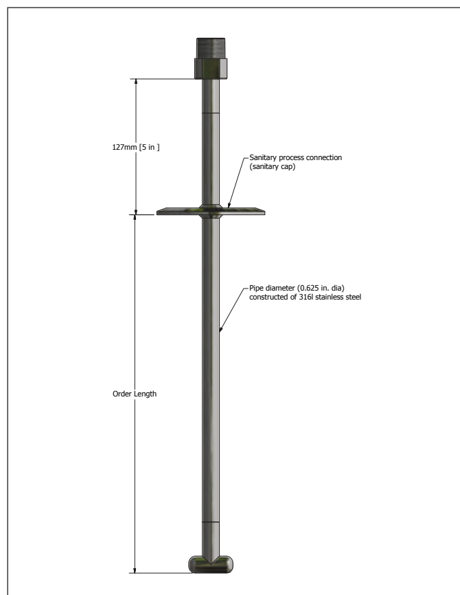
Fig. 5: Configuração da haste externa
