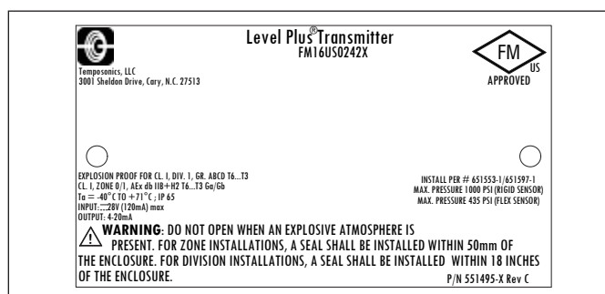
Fig. 25: À prova de explosão, etiqueta FM, HART®, invólucro opções G, H ou L
