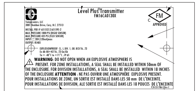
Fig. 42: À prova de explosão, etiqueta FMC, Modbus ou DDA, invólucro opções D, E
