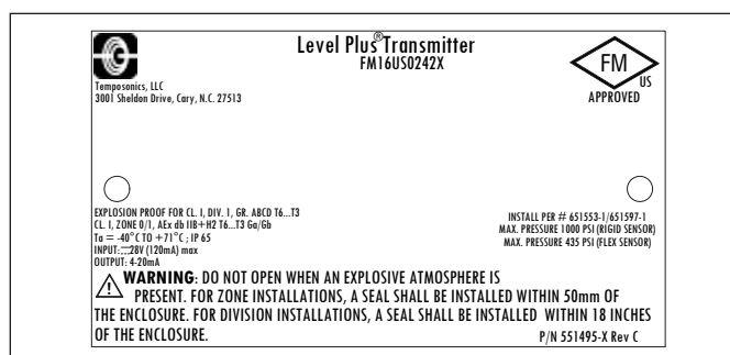
Fig. 26: À prova de explosão, etiqueta FM, HART®, opções de invólucro D, E
