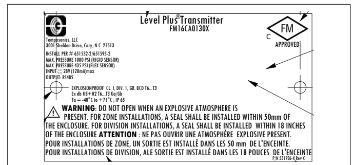
Fig. 43: À prova de explosão, etiqueta FMC, HART®, invólucro opções G, H ou L
