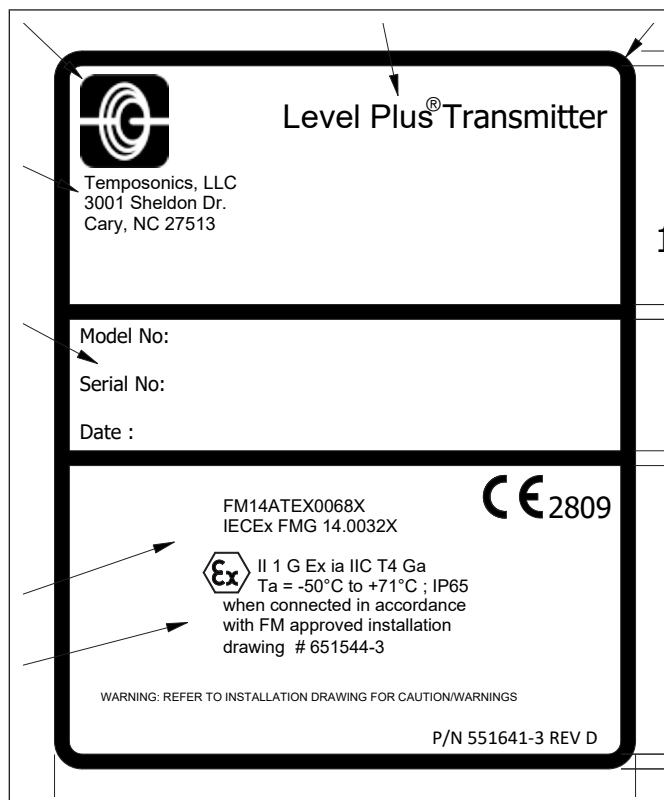
Fig. 52: Etiqueta ATEX/IECEX intrinsecamente segura, Modbus e DDA, invólucro NEMA
