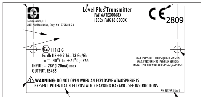
Fig. 59: À prova de chamas, etiqueta ATEX e IECEx, invólucro Modbus ou DDA, opções D, E, G, H ou L
