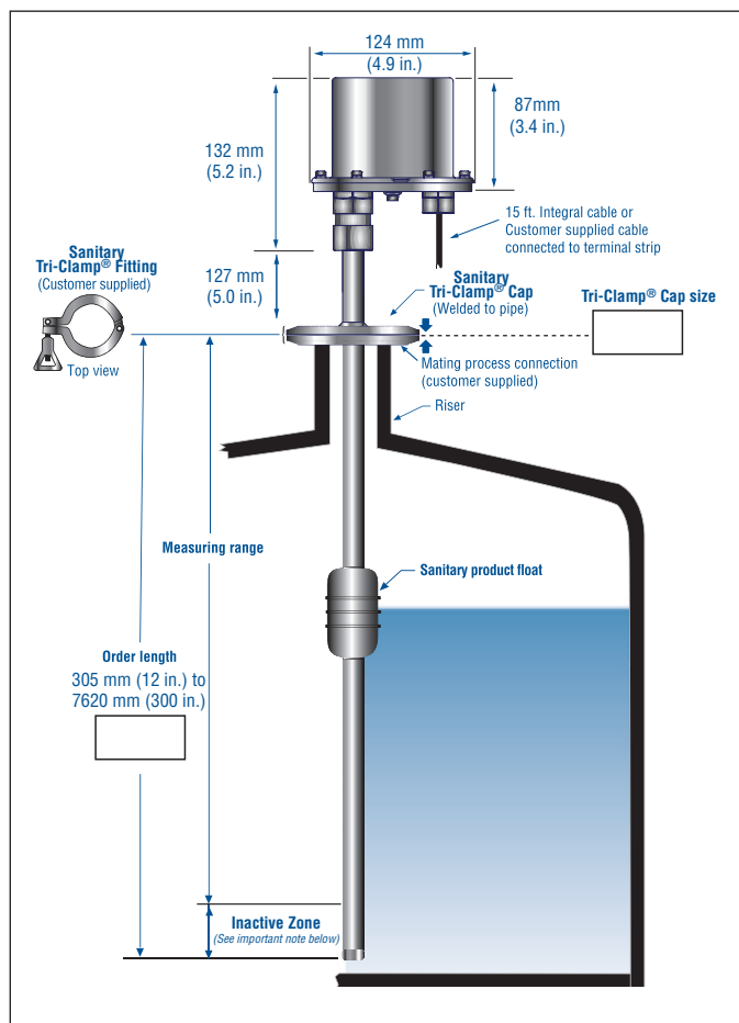
Fig. 9: Montagem da haste com braçadeira Tri-clamp
